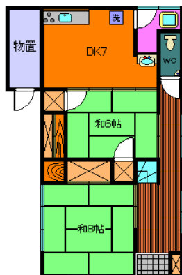
1階
