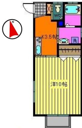
《間取り》
