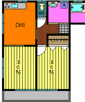
《配置図》
